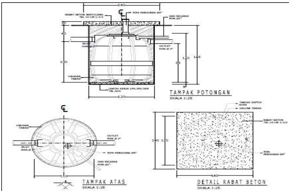
Gambar 4.19 Tangki Pabrik
