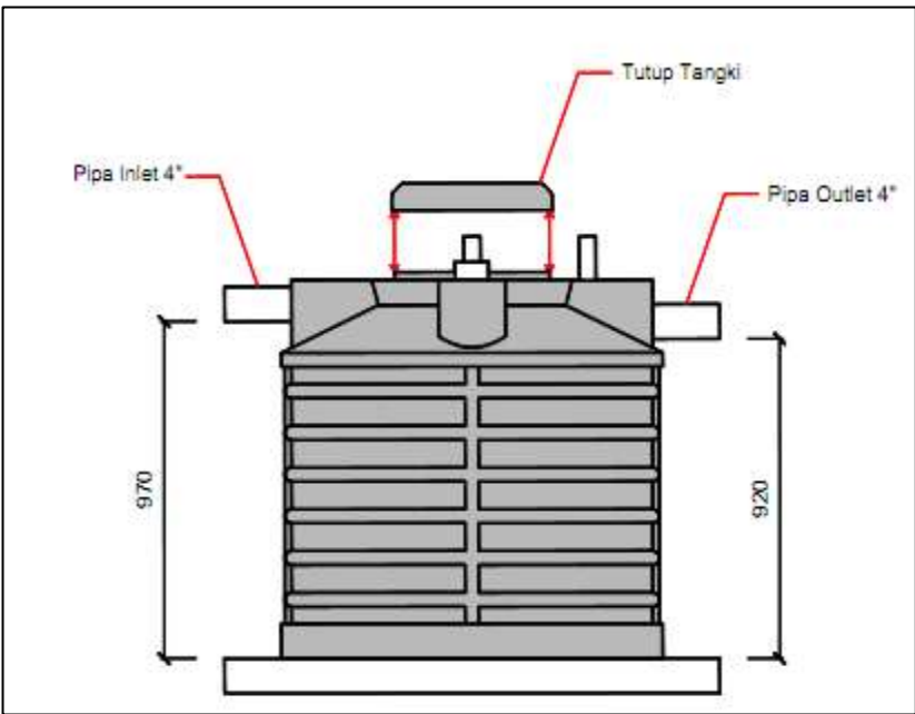
Gambar 4.20 Tangki Pabrik 0,6
