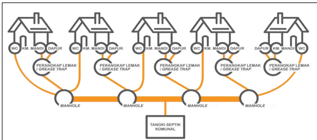
Gambar 4.13 Ilustrasi Tangki Septik Komunal (5-10 KK)
